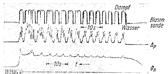
Abb. 6. Meßergebnisse von Pulsationen für einen Systemdruck von 1 bar.
