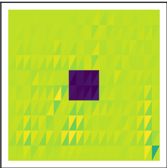
MAP \psi^*
