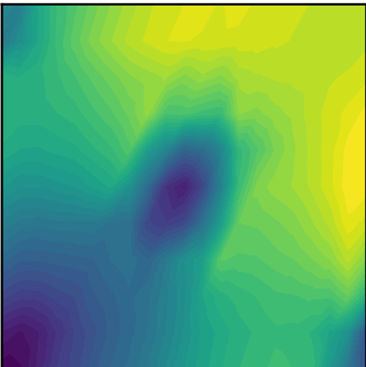
MAP \psi^*
